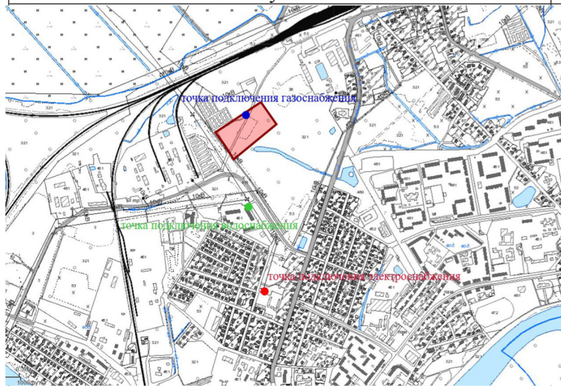
план участка
